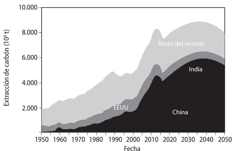
Figura 8.6: Extracción de carbón y proyección futura (Li, 2017).
