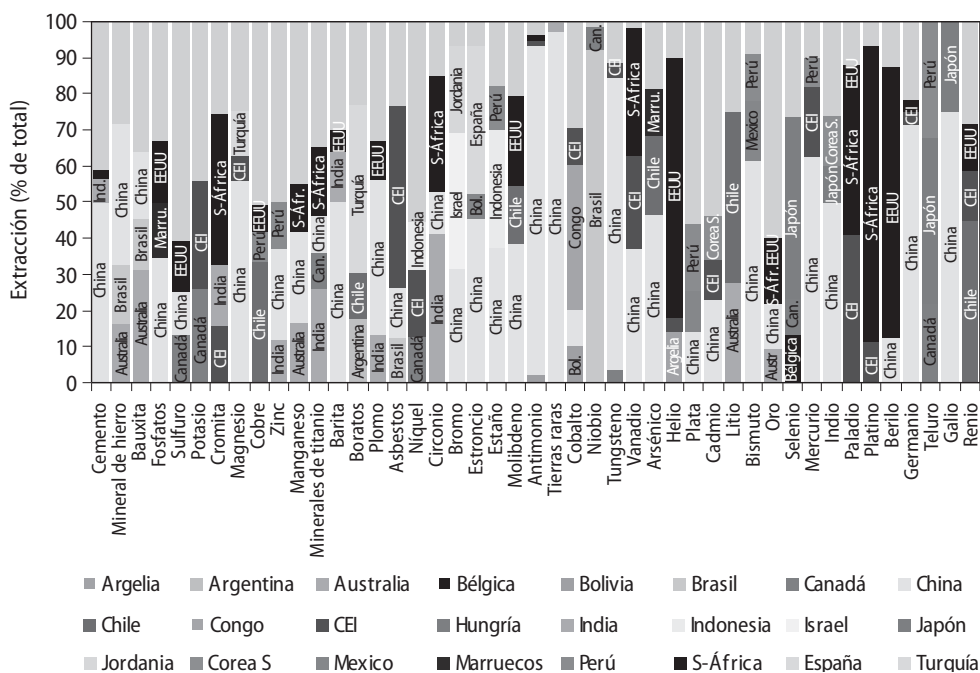
Figura 9.12 Extracciones de distintas materias primas por países en 2009 (Zittel, 2012).
