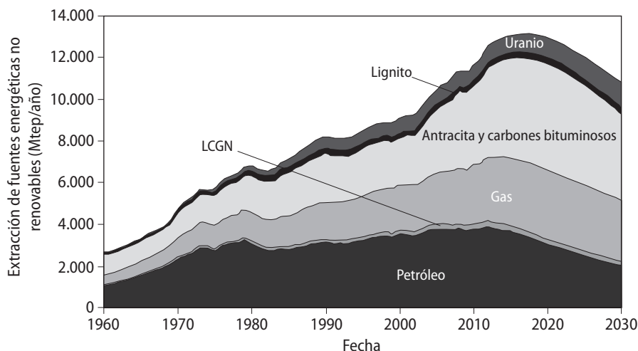
Figura 8.7 Disponibilidad de fuentes energéticas no renovables y proyección futura (Zittel y col., 2013).
