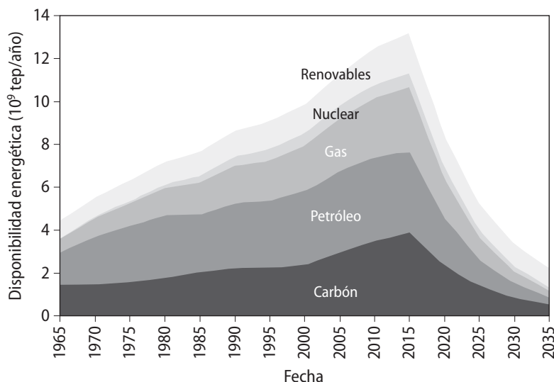
Figura 9.7 Estimación de la disponibilidad de energía futura (Tverberg, 2014g).
