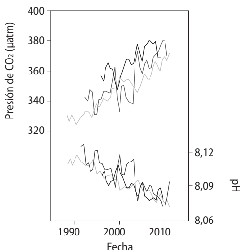
Figura 8.18 Concentración de \text{CO}_2 en la superficie oceánica y pH (IPCC, 2013).
