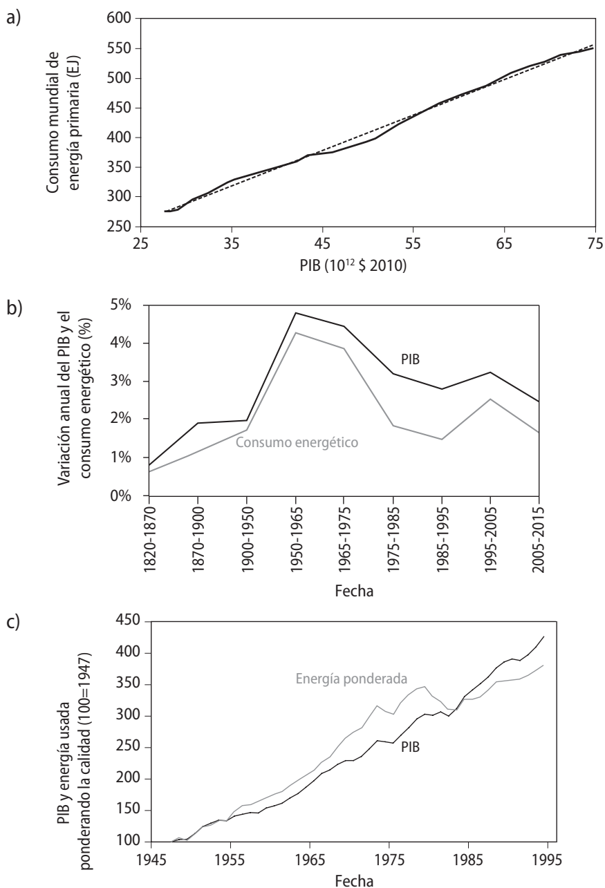
Figura 8.24 a) Correlación entre el consumo de energía primaria y el PIB real a nivel mundial entre 1980 y 2015 (Coyne, 2016). b) Variación del PIB mundial y del consumo de energía (Tverberg, 2015b). c) PIB de EEUU en dólares constantes frente a la calidad de la energía usada. Este índice pondera los pesos de cada tipo de energía y sus precios (Stern, 2004).
