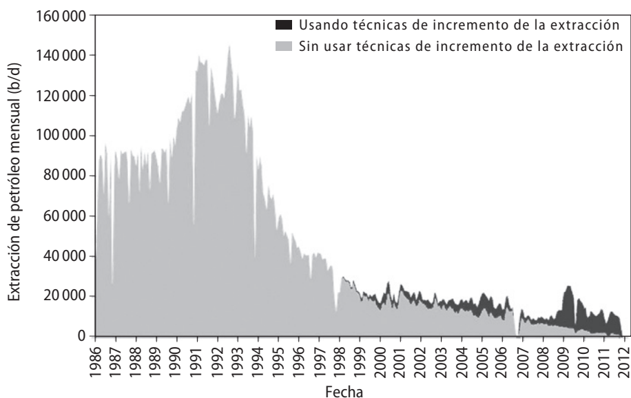
Figura 8.3 Extracción de crudo de los campos Magnus (a) y Ula (b) sin usar técnicas de incremento de la extracción y utilizándolas (Muggeridge y col., 2013).
