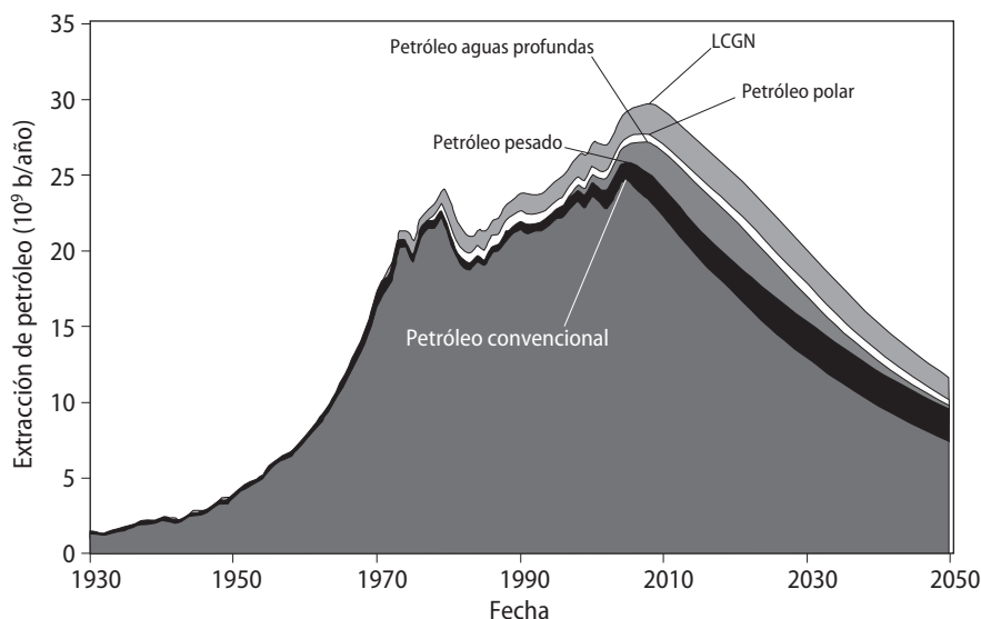
Figura 8.4 Extracción de petróleo y proyección futura 340 (Heinberg, 2012).
