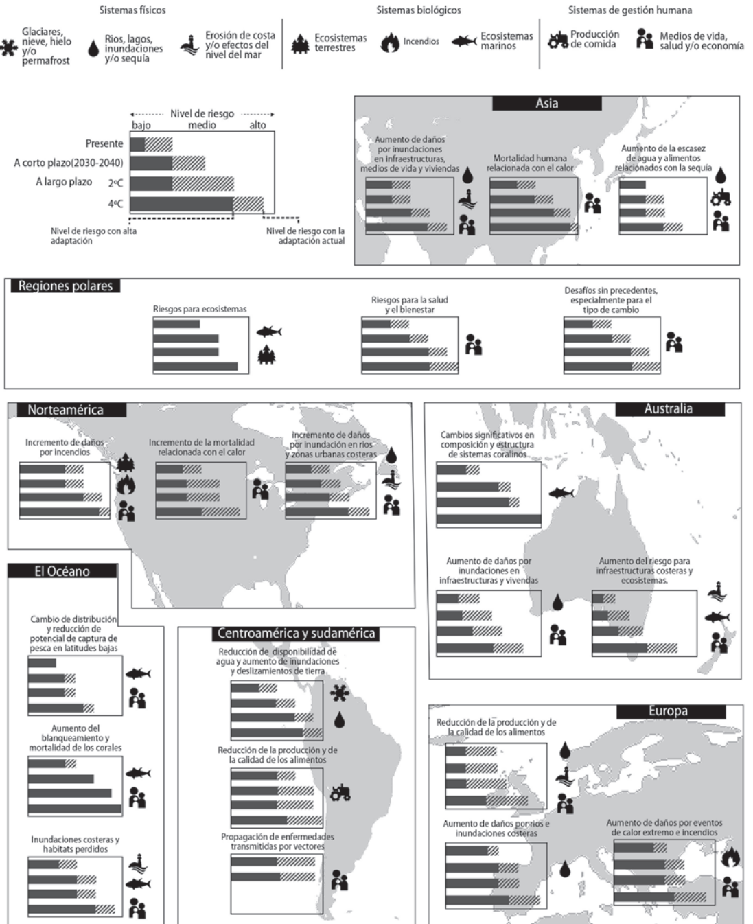
Figura 9.13 Impactos del cambio climático por regiones (IPCC, 2014a).
