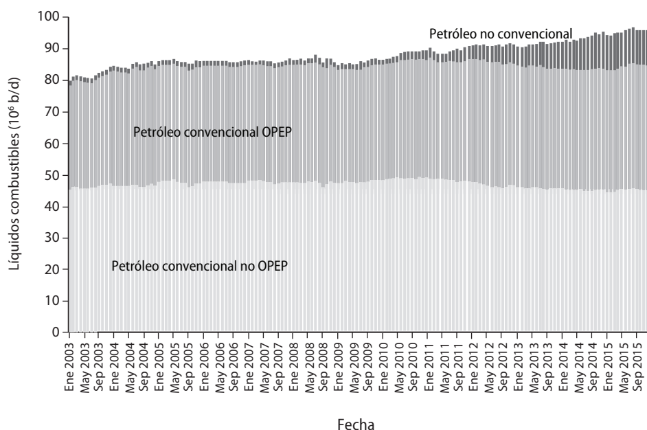
Figura 8.1 Extracción de petróleo mundial (Berman, 2015).
