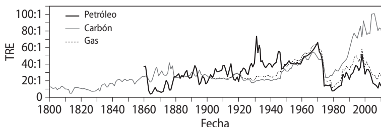
Figura 8.8 a) Relación entre la TRE y la energía neta (Morgan, 2013). b) TRE del carbón, gas y petróleo (Court y Fizaine, 2016).
