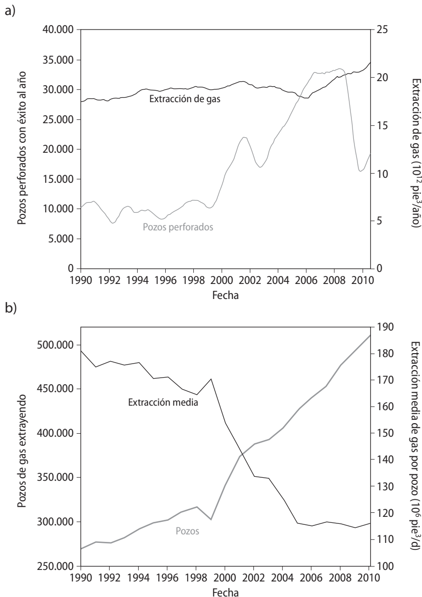
Figura 8.12 a) Extracción de gas natural en EEUU y número de pozos perforados con éxito. b) Número de pozos en funcionamiento y rendimiento por pozo en EEUU (Hughes, 2011).
